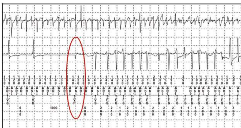
Рисунок 1: Внутрисердечная электрограмма с эпизодом желудочковой тахикардии, возникшим после эффективной стимуляции желудочков.
